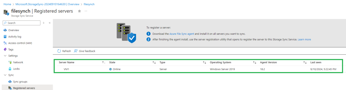
Рисунок 4. Зареєстрований сервер додано до компонента Azure File Synch Agent в Azure Resource Manager.
