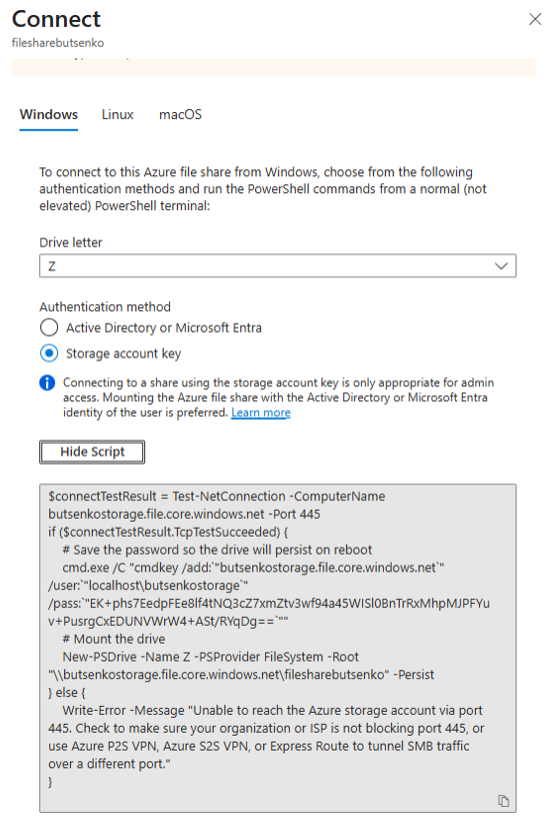
Рисунок 3. Генерація ключа для встановлення зв'язку між папками з файлами на локальному диску та в хмарі
