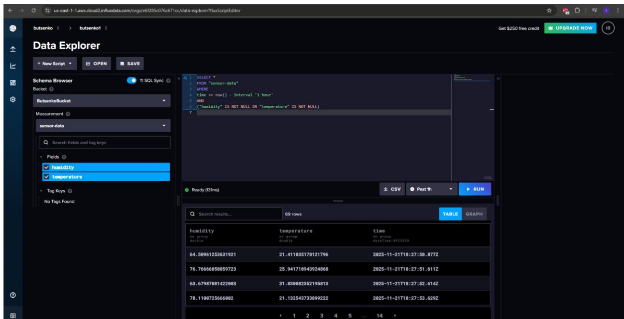
Рисунок 4. Дані приладу IoT, збережені в таблиці InfluxDB.
