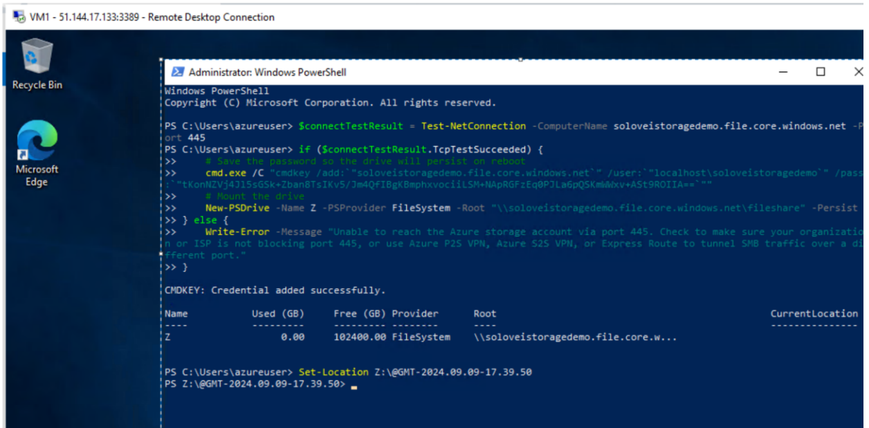
Рисунок 4. Інсталляція ключа на віртуальній машині.
